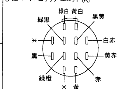
S-02 ハイドロリック・ユニット (A)
