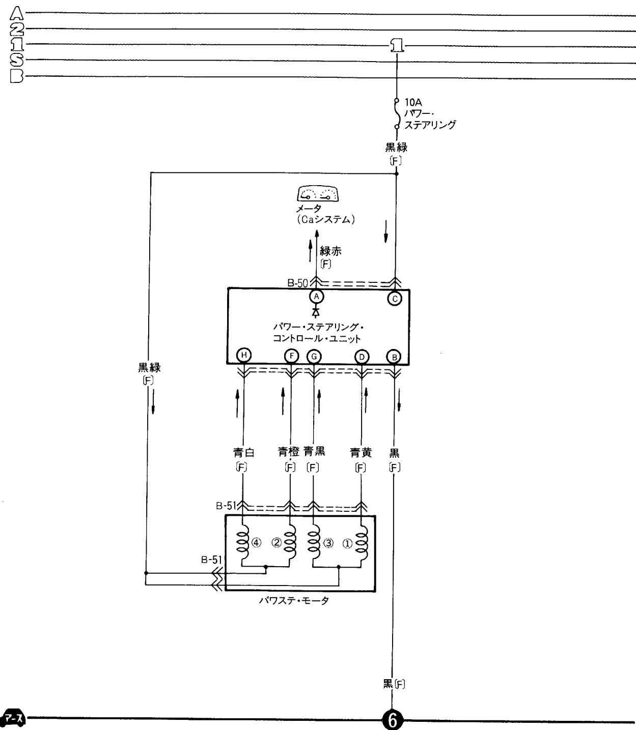
B-50 パワー・ステアリング・コントロール・ユニット(F)
